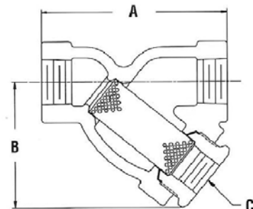
Corte Filtro "Y" 1/2" - 2"
